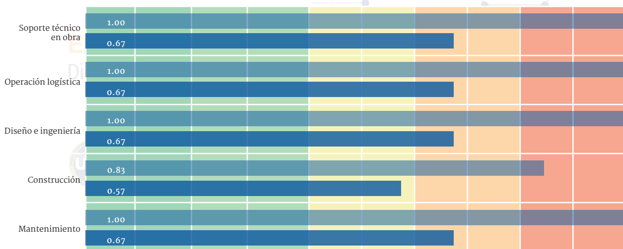
Gráfico 63. Resultados de vulnerabilidad inherente al LA Obras de Ingeniería Civil.
